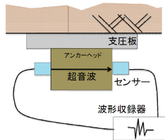
超音波を用いたグラウンドアンカーと施工アンカーボルトの調査システム
