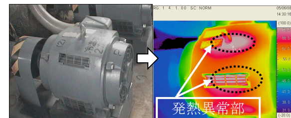
「赤外線カメラ」を用いた点検精度向上
