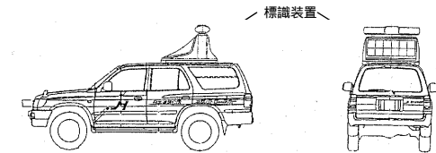
道路巡回車(A 1)の構成
