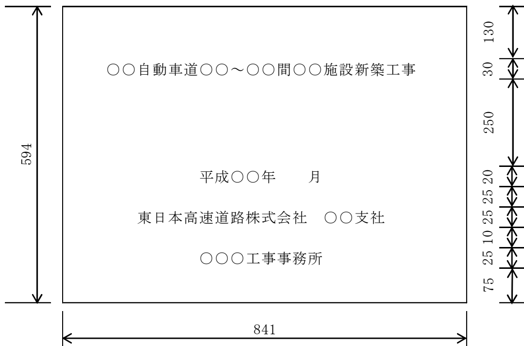
図－３ 表 紙
