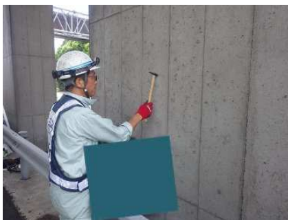
目視、打音検査
