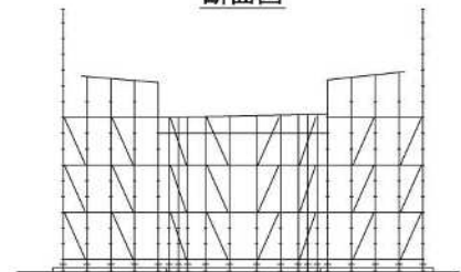
断面図
