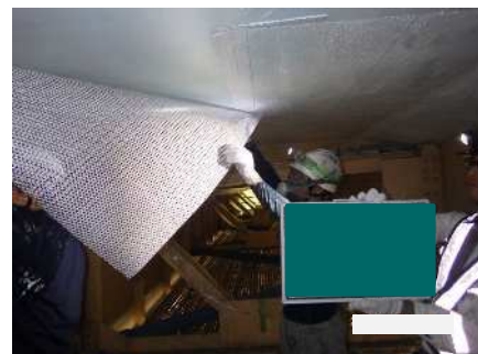
④連続繊維シート接着
