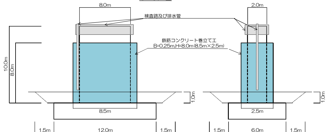
形 状 図
