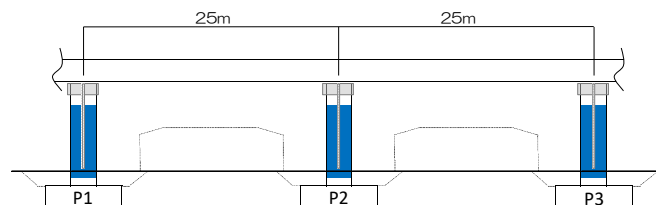
橋脚配置図
