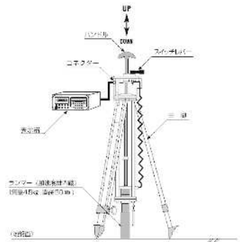
簡易支持力測定器 (キャスボール)
