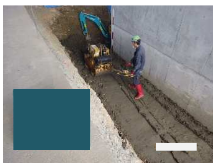
埋戻し・締固め
