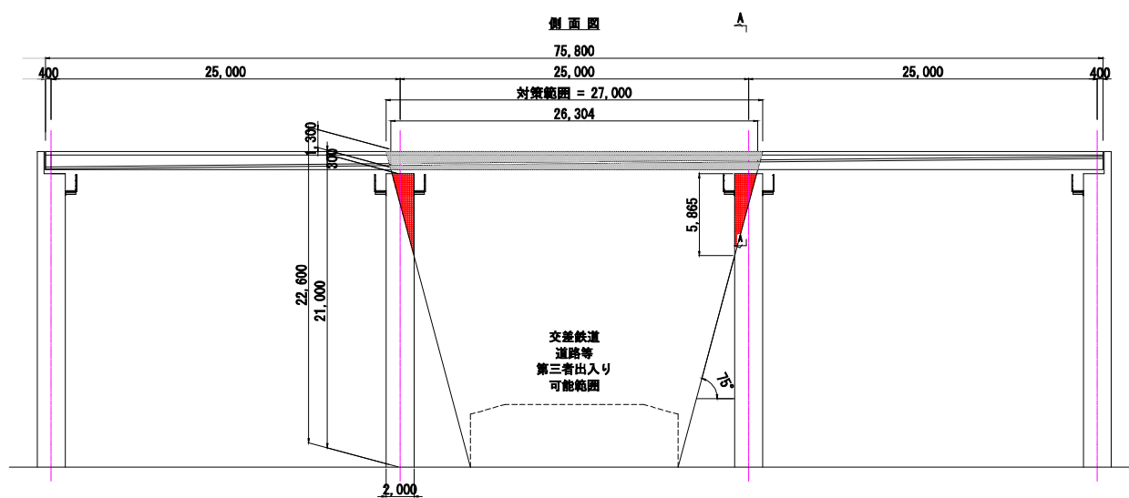
数量算出用の構造図
