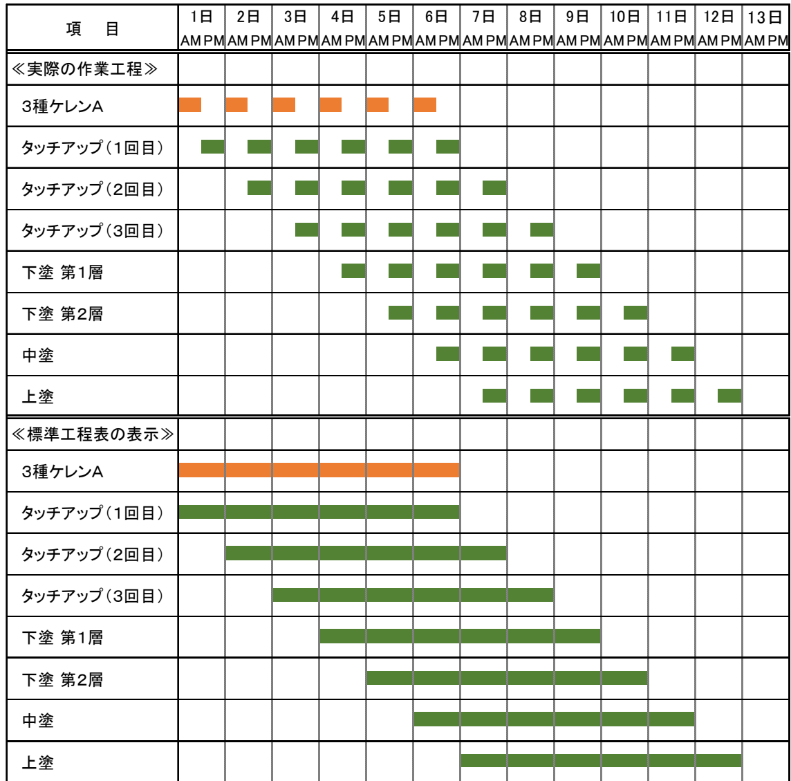
図 5-14-6 塗装面積 500 ㎡当たりの 3 種ケレン～塗装作業までの施工工程（概念図）
