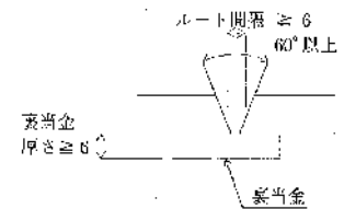
現場継手形状
