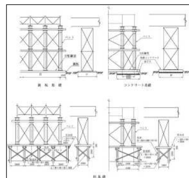
ベント基礎の種類
