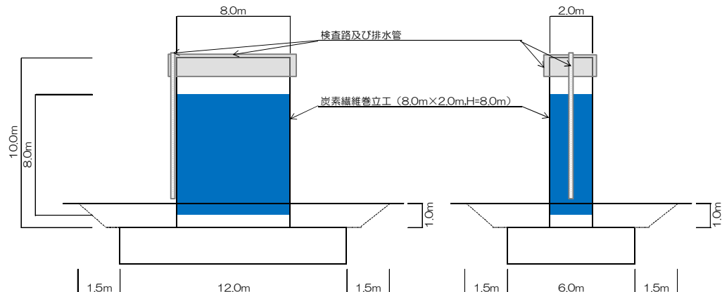
数量算出用の構造図
