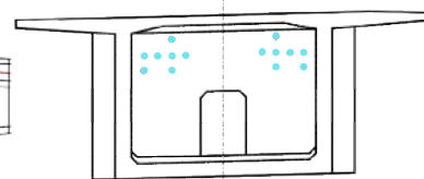
柱頭部断面
