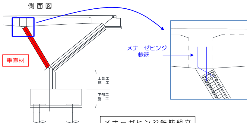
メナーゼヒンジ鉄筋 (亜鉛メッキ処理)
