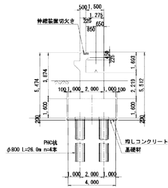
側面図
