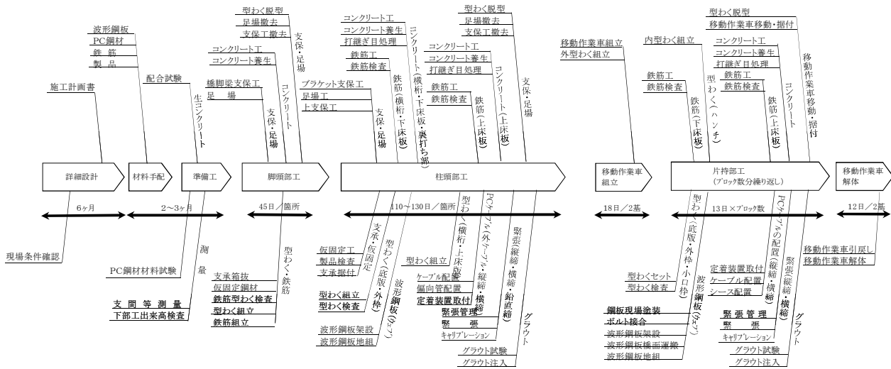
PC橋（片持ち架設工法による波形スラブ橋桁橋）工事施工の流れ
