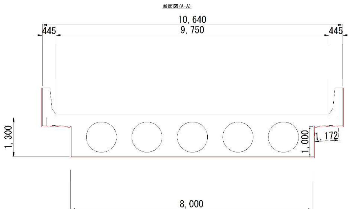
数量算出用の構造図
