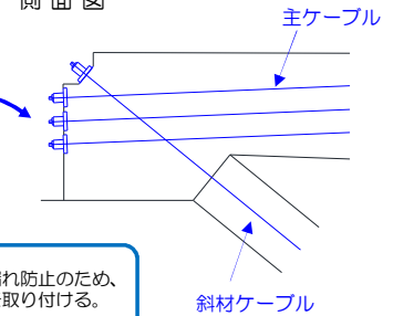
側面図
