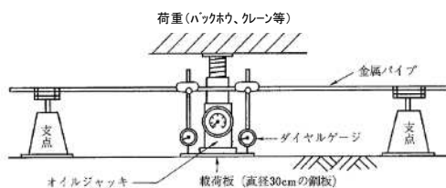
平板荷重試験
