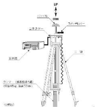
簡易支持力測定器(キャスボル)
