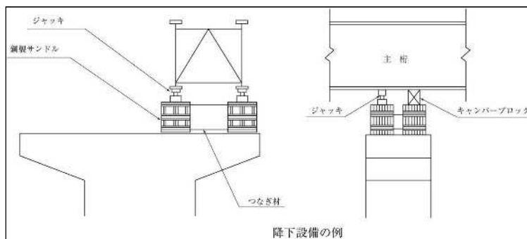
降下設備の例
