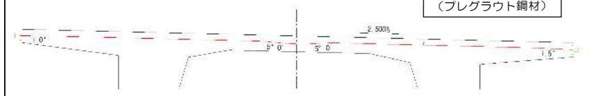
床版横締めケーブル形状図
