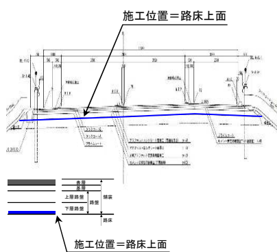
図一標準横断面図
