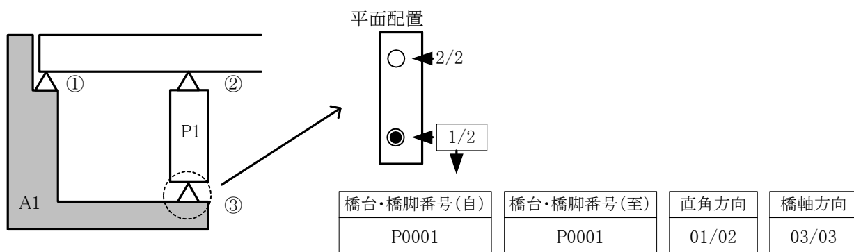
(d) ロッカー橋脚下側支承の場合
