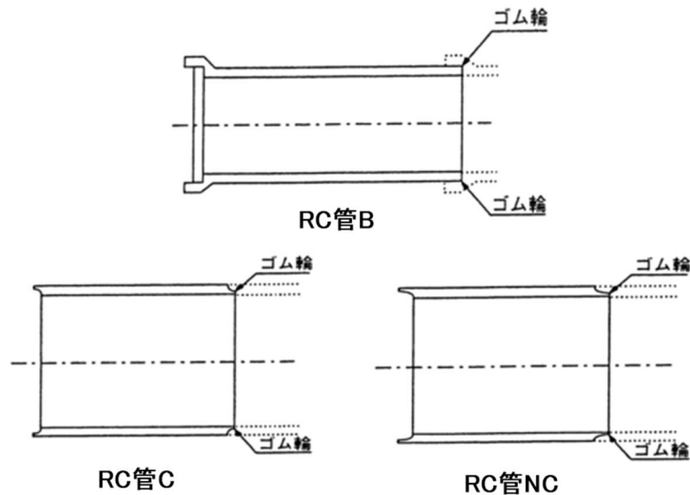
プレストレストコンクリート管の継手の構造、特性
