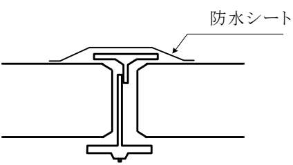
II-B型(側壁)
