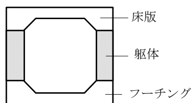
(5) ボックス橋
