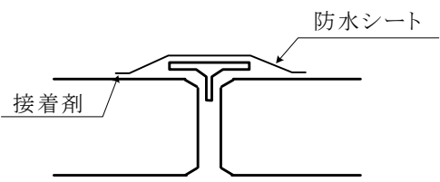
II-A型(頂版)
