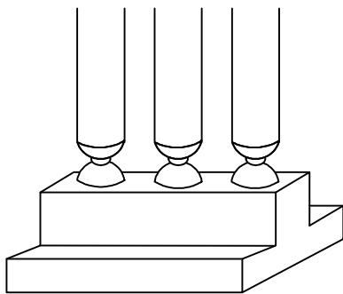
柱式ロッキング橋脚
