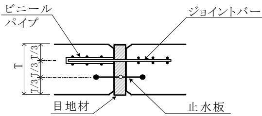
III型(底版)
