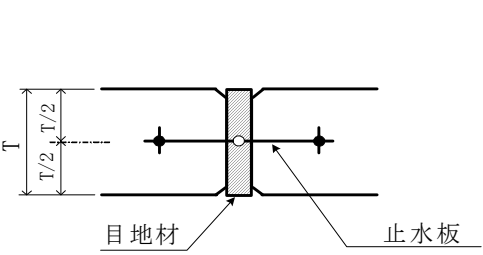
I 型
