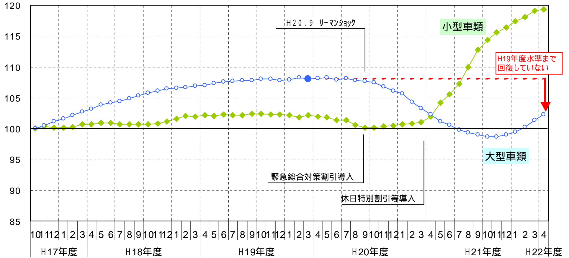
高速道路走行台 千 の推移 (12ヶ月移動和、H17.10 = 100)
