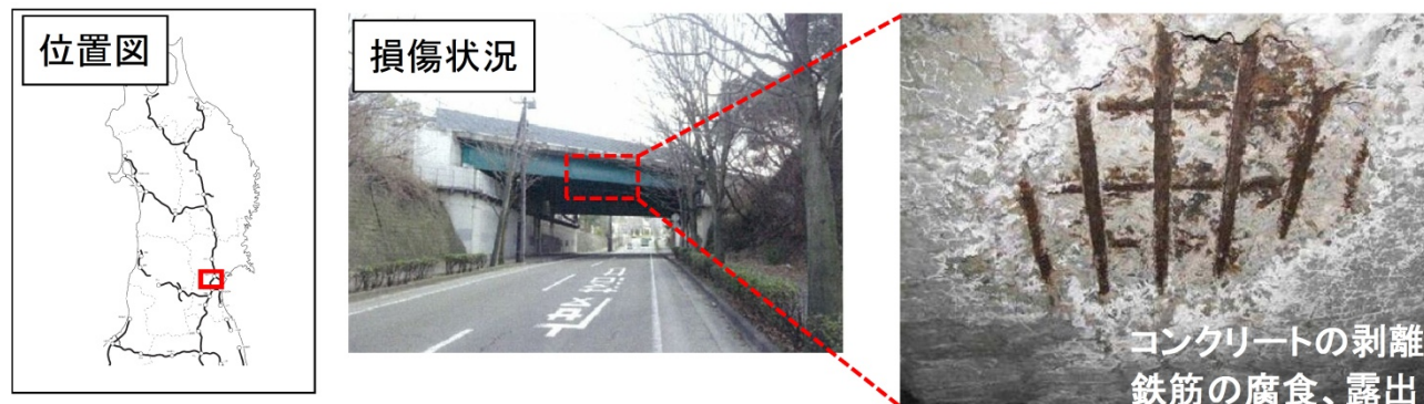
写真1 東北自動車道（仙台宮城 IC～泉 IC 間）中山橋
