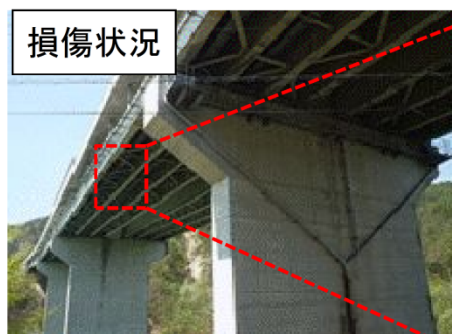
写真2 長野自動車道（安曇野 IC～麻績 IC 間）小仁熊橋
