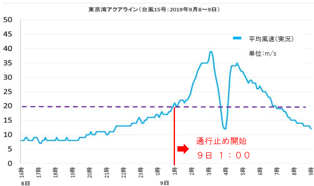
図2 台風15号接近時の東京湾アクアラインの風速
