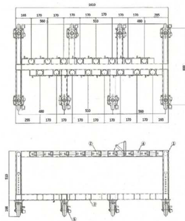
標識用土台 参考図
