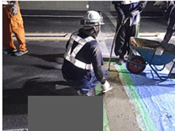
伸縮装置補修状況
