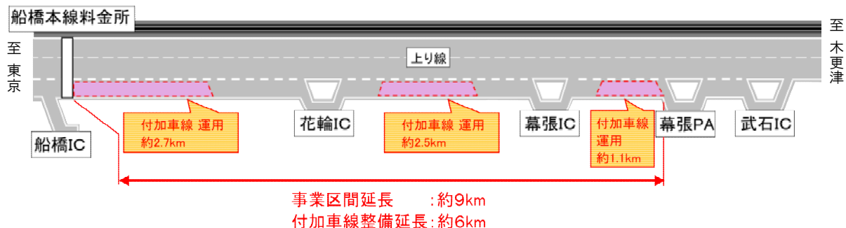
【対策前】
