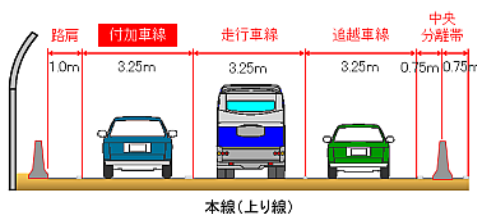
【対策後】
