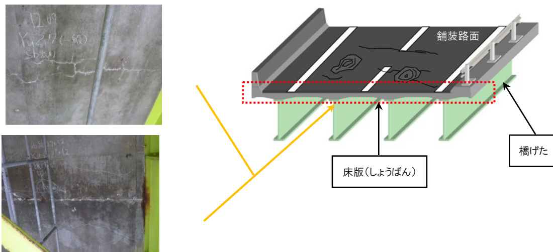
【床版下面のコンクリートひび割れ状況(夕張川橋)】
