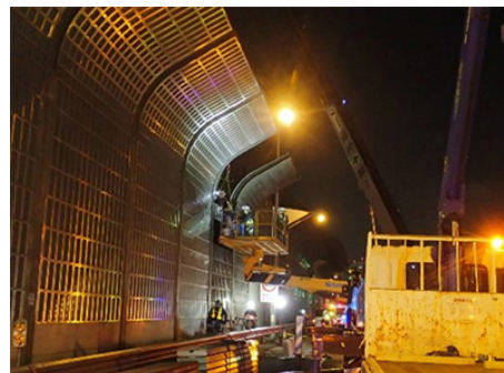
遮音壁補修工事 作業状況
