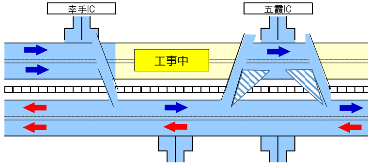
今回 (2)車線運用切替(幸手IC～五霞IC)【8月29日5時以降の車線運用】
