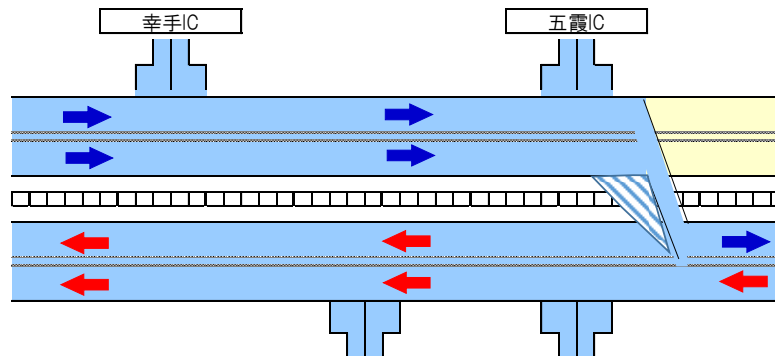
(4)(参考)今後の車線切り替え②(幸手IC～五霞IC4車線化済)
