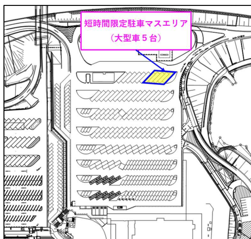
図-3 佐野SA(下り)整備状況(5マス)
