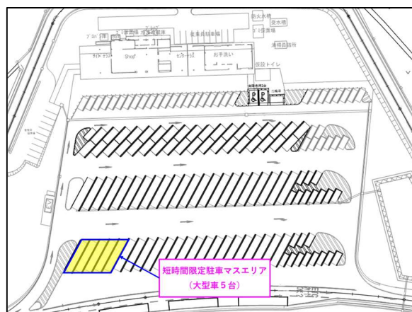
図-5 狭山PA(外回り)整備状況(5マス)
