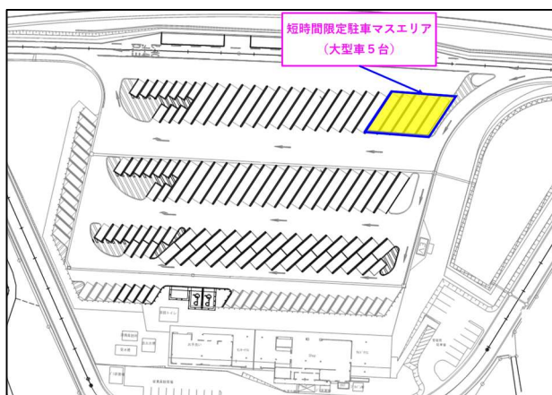
図-4 狭山PA(内回り)整備状況(5マス)
