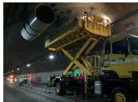
施設保全点検（トンネル点検）例
