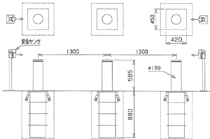
《装置概要(ボラード)》
