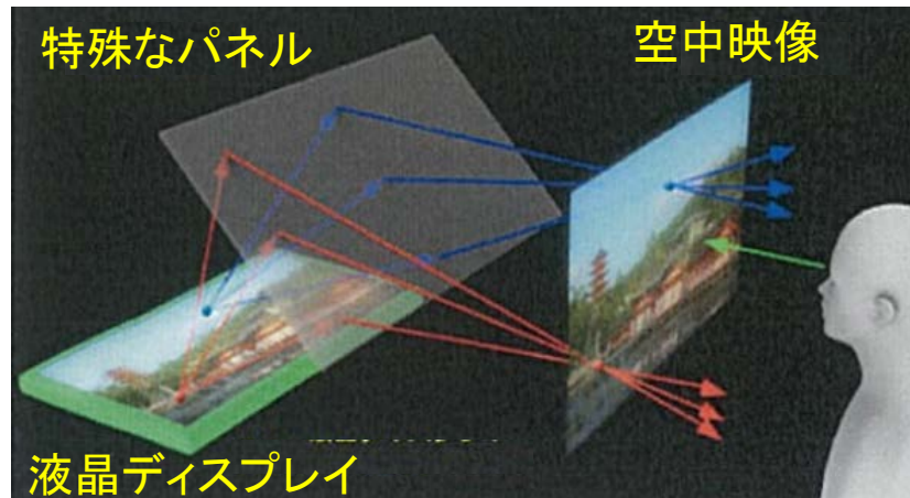
《原理》
