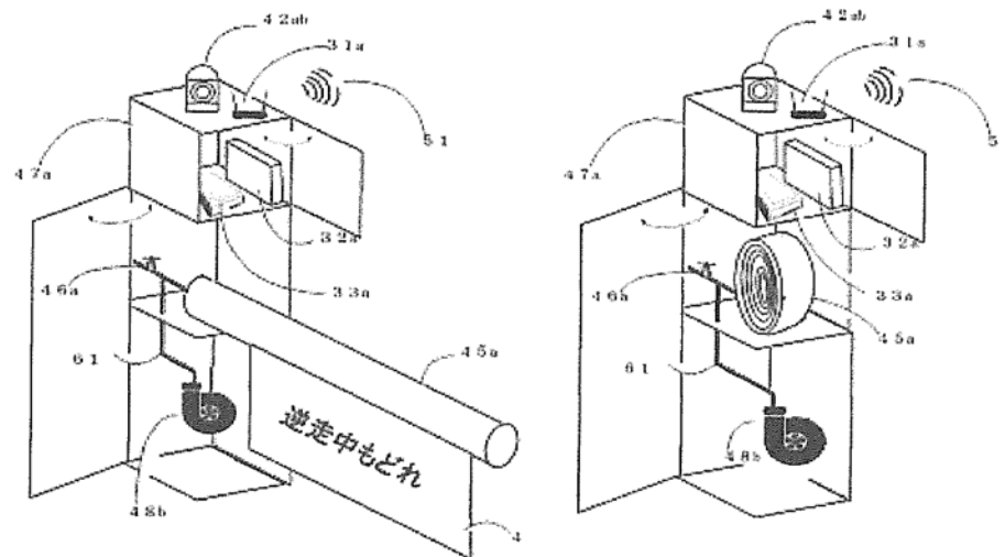
《装置概要》
