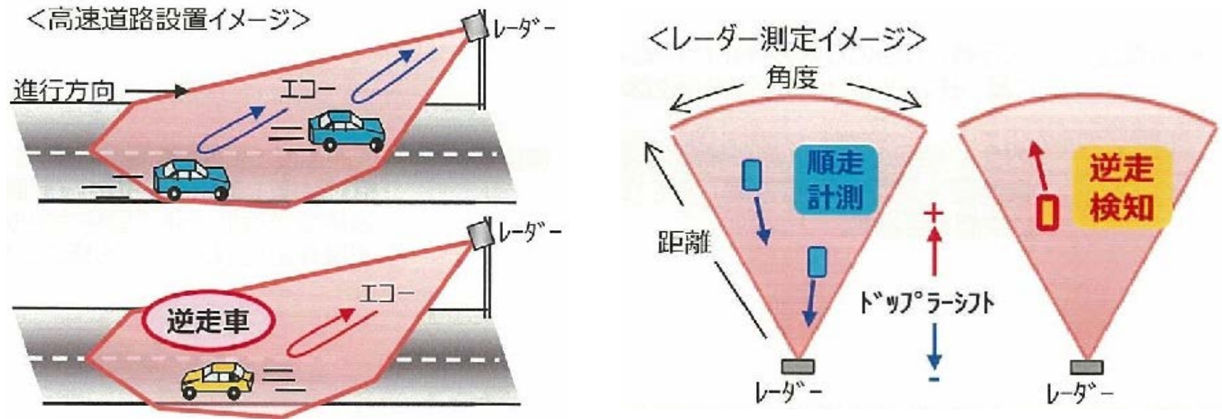
《ドップラーレーダーによる車両検知イメージ》
