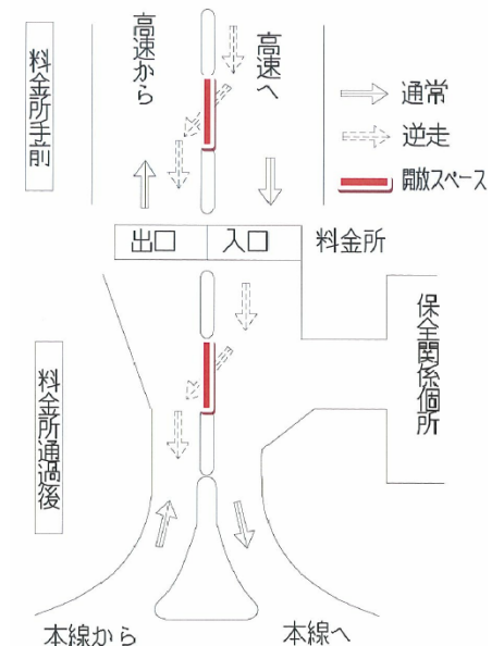
《設置箇所イメージ》
