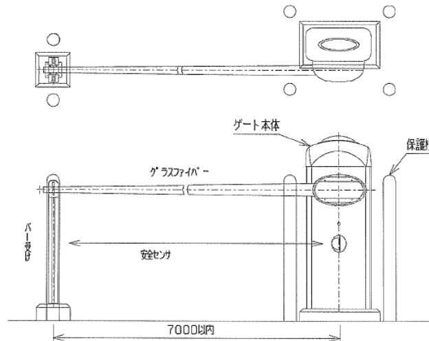
《装置概要(バーゲート形式)》
