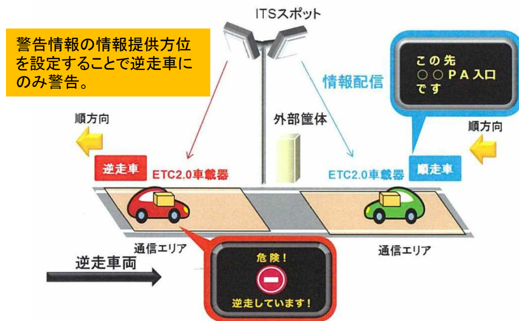
《提案技術のイメージ》
