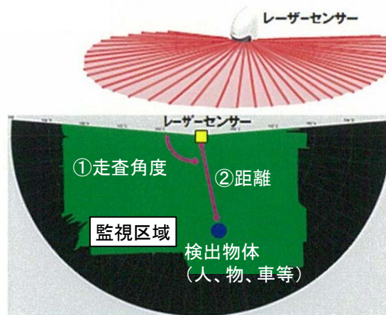
①走査角度、②距離の情報から 物体の位置を検出
