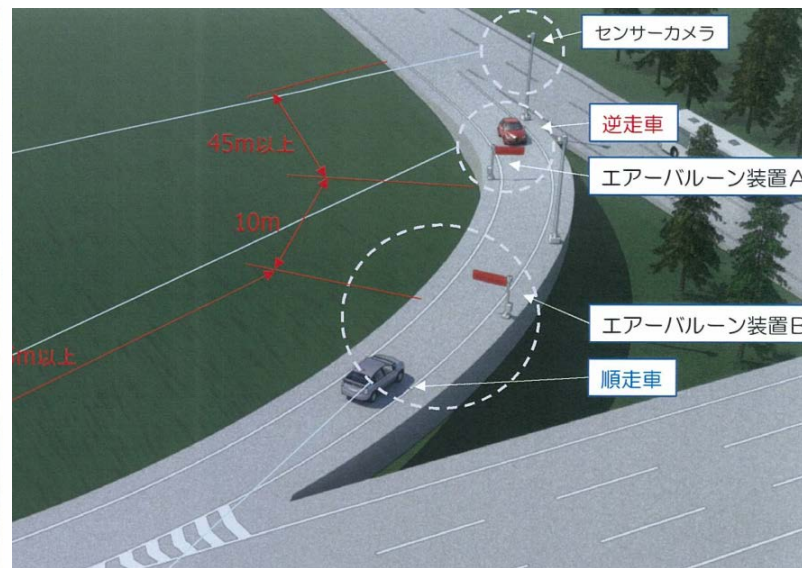
①センサーによる逆走検知
