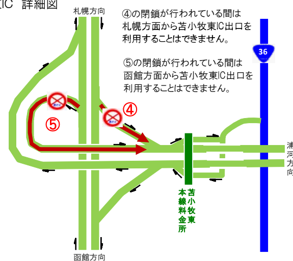
苫小牧東IC 詳細図
