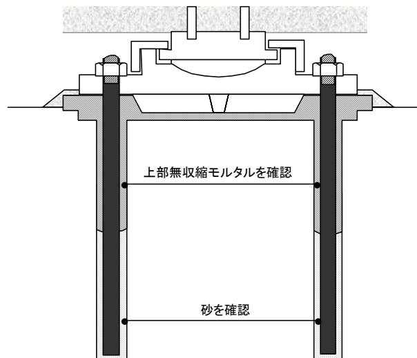
支承詳細図(正面図)
