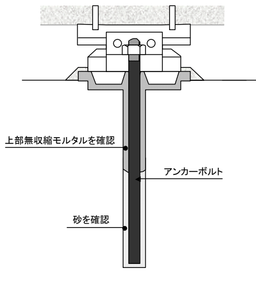
支承詳細図(断面図)
