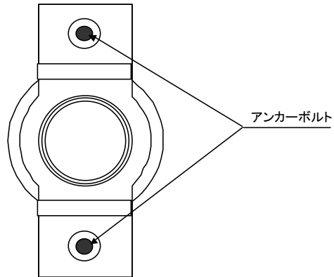
支承を上から見た図
