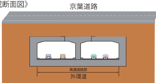
《完成断面図》
