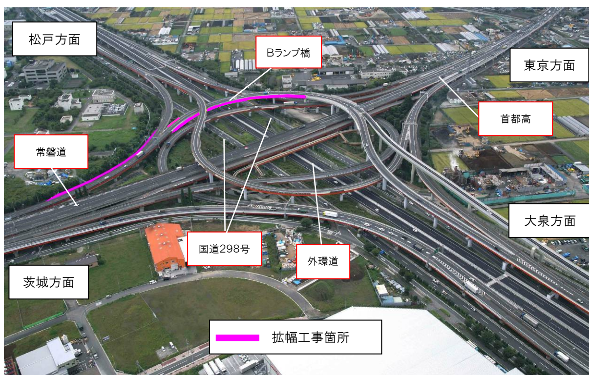
三郷JCT架設概要図
