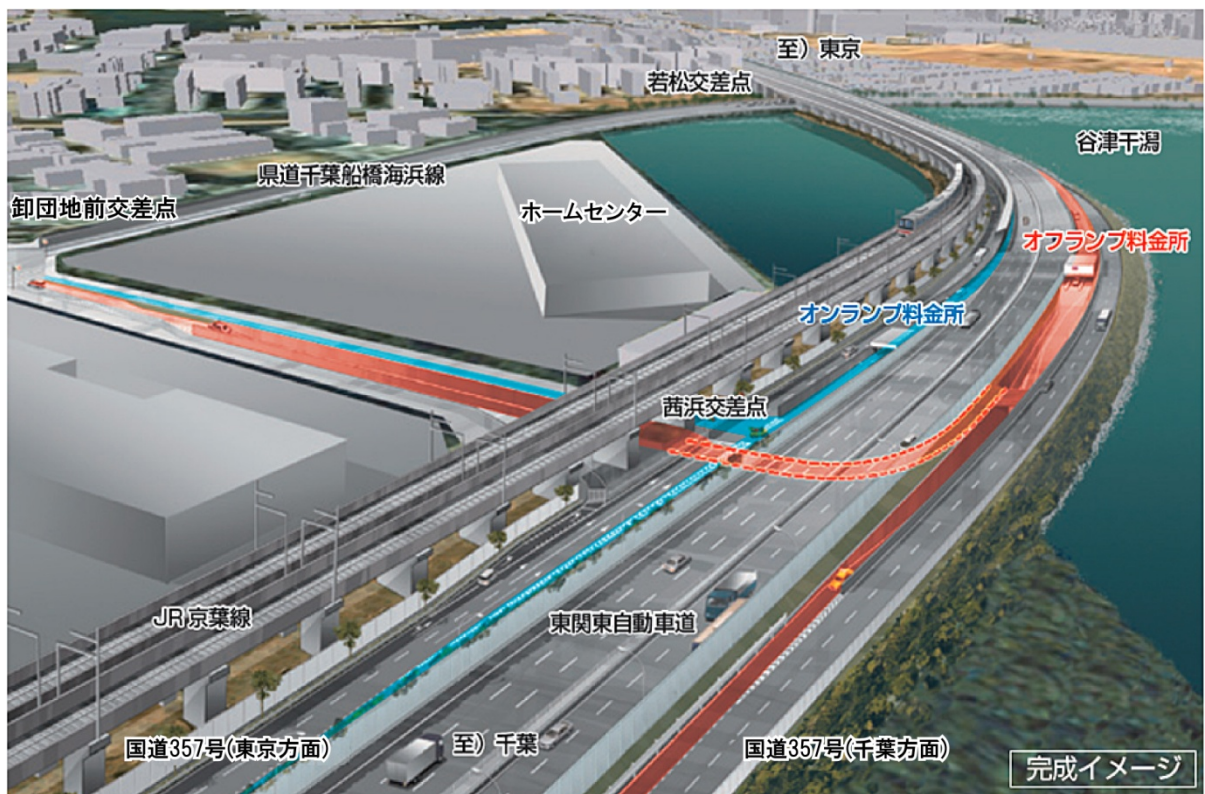
谷津船橋インターチェンジ完成イメージ図
