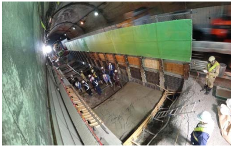
② 掘削～型枠～コンクリート打設
