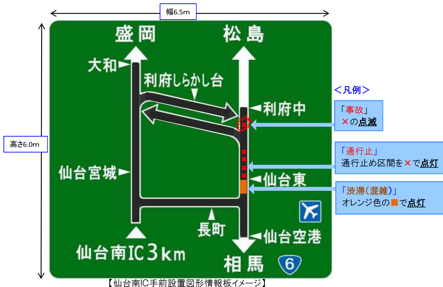
【図形情報板の表示概要】
