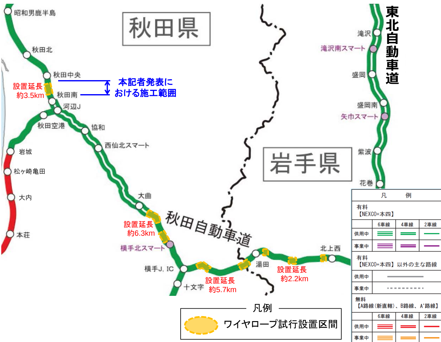
試行設置区間図
